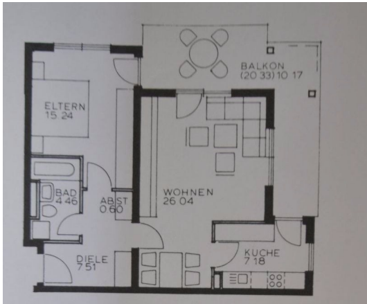
Grundriss
