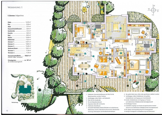
Grundriss Planung1
