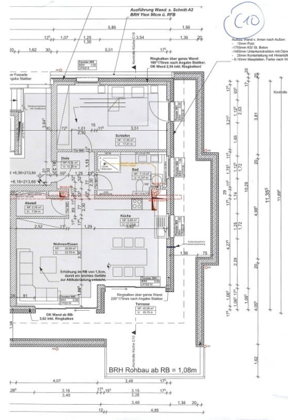
Grundriss
