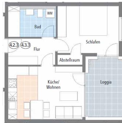
Grundriss 4.2.3.
