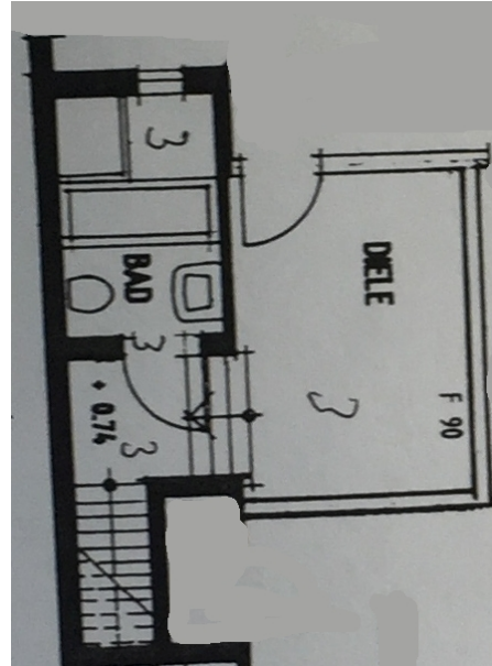
Grundriss EG
